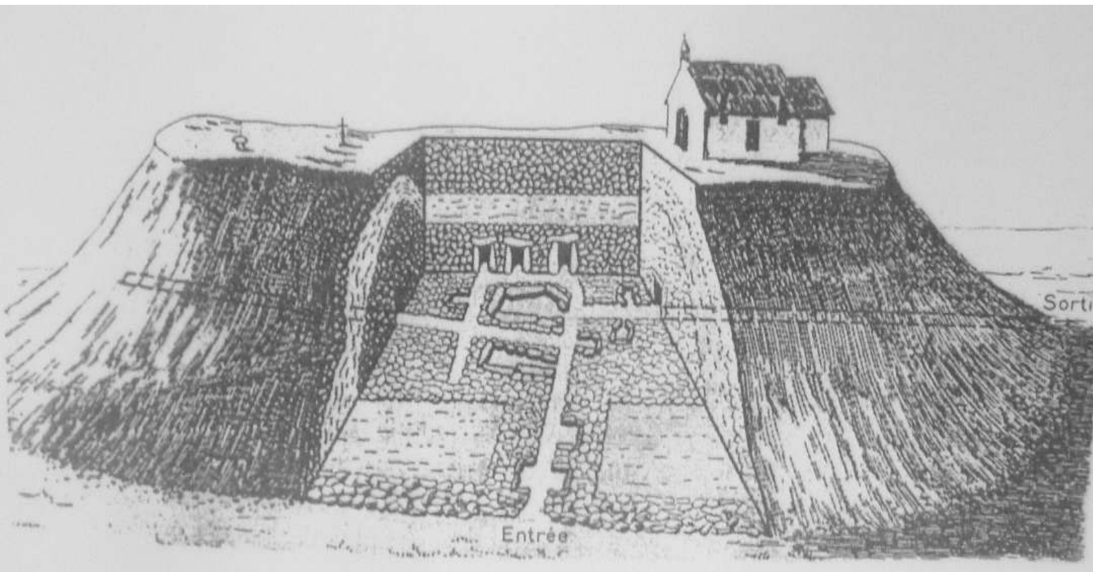
Vue en coupe du tumulus.
